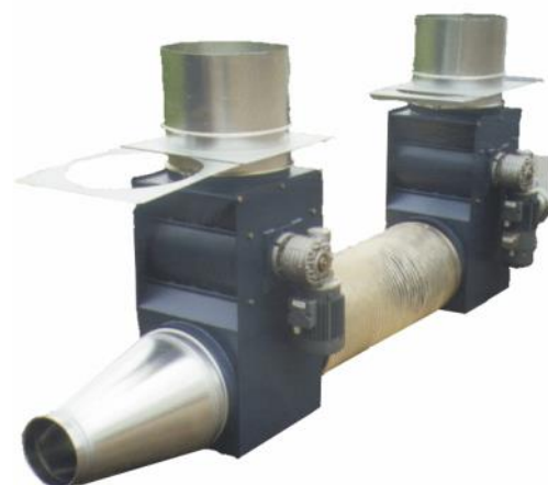
STYROMETER unidad de mezcla para asegurar una mezcla exacta de material reciclado EPS y perlas nuevas justo delante el molde de bloque. Ya sea directamente al molde de bloque o al silo de alimentación del molde de bloque. También para mezclar materiales EPP delante el tanque de pre-presurización.
