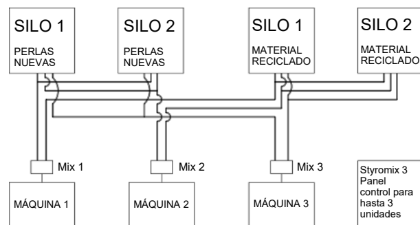
Panel de control para 3 unidades de mezcla individuales para 3 máquinas.
